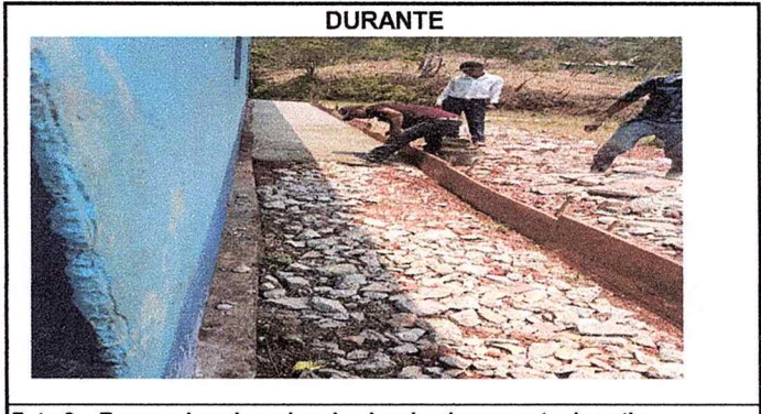
Foto 6: Empezo la colocacion de plancha de concreto de patio.
